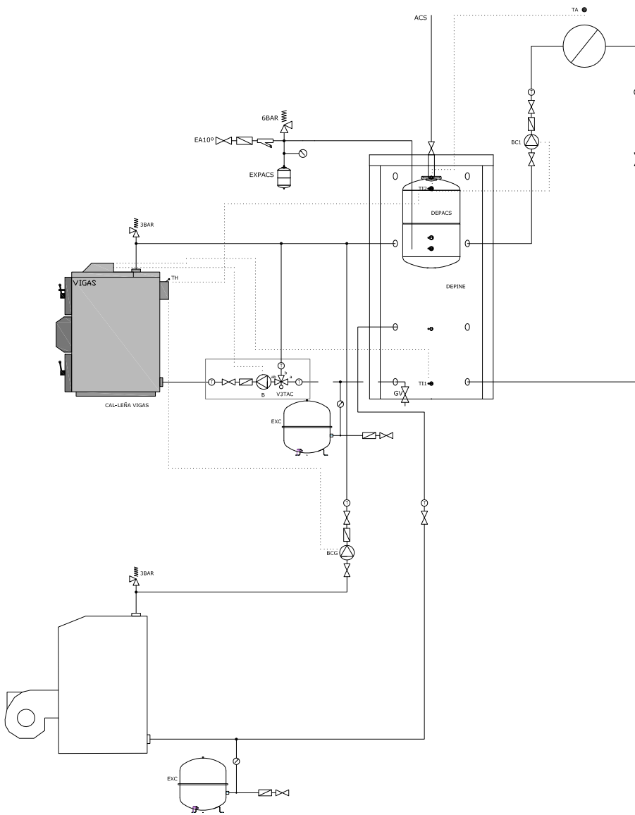
CALEFACCION Y ACS CON GAS-GASOLEO E INERCIA DEPOSITO KOMBI
