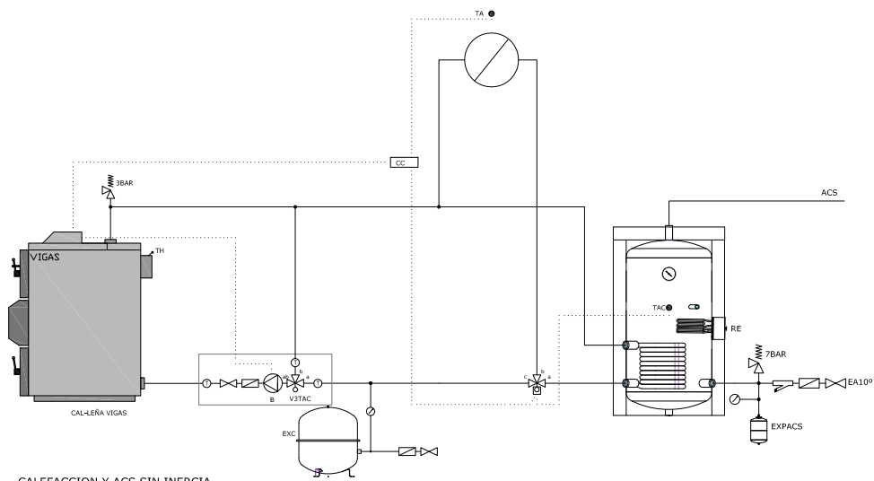
CALEFACCION Y ACS SIN INERCIA
