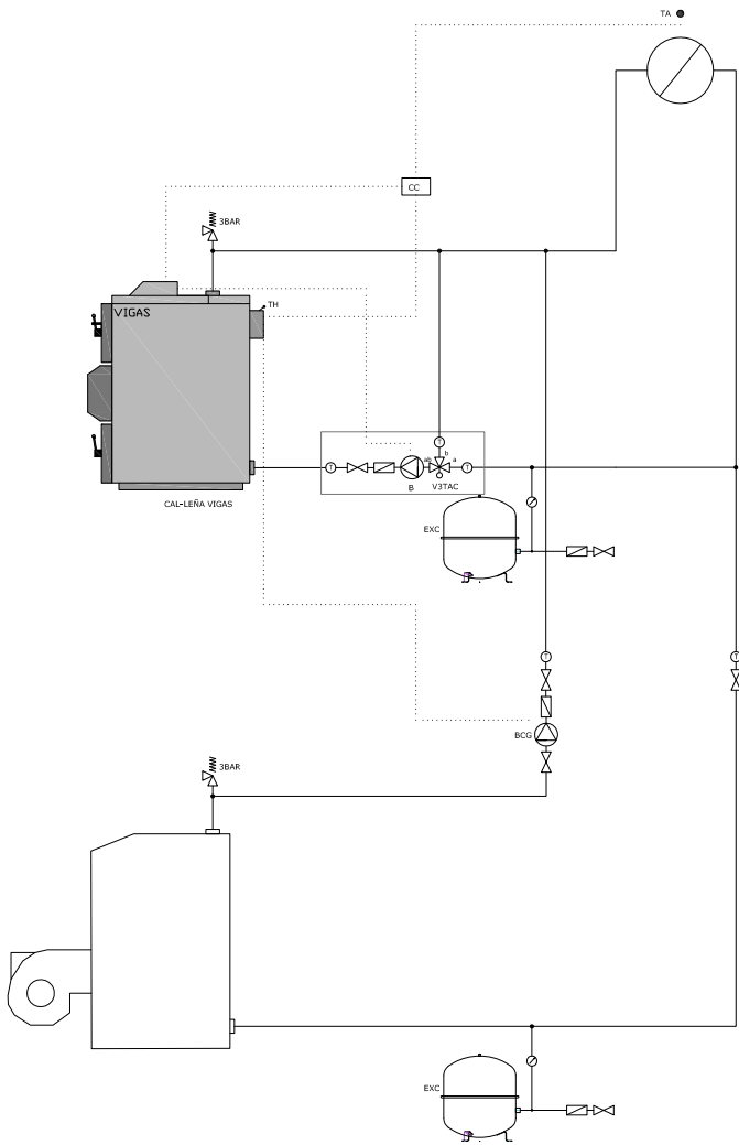
SOLO CALEFACCION COMBINADO CON GAS-GASOLEO
