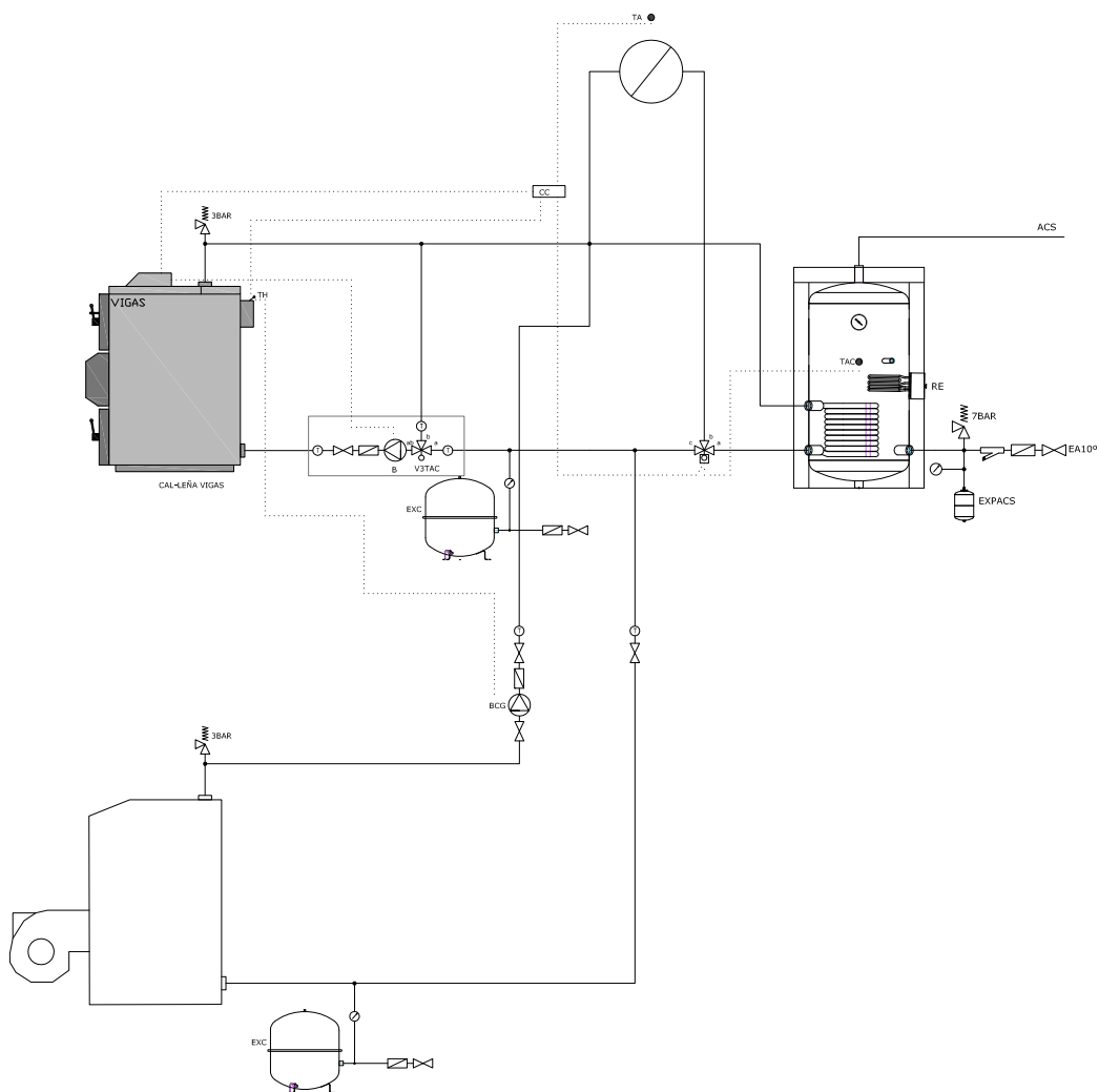
CALEFACCION Y ACS EXTERIOR CON CALDERA DE GASOLEO
