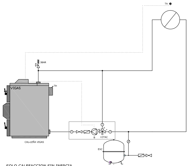
SOLO CALEFACCION SIN INERCIA
