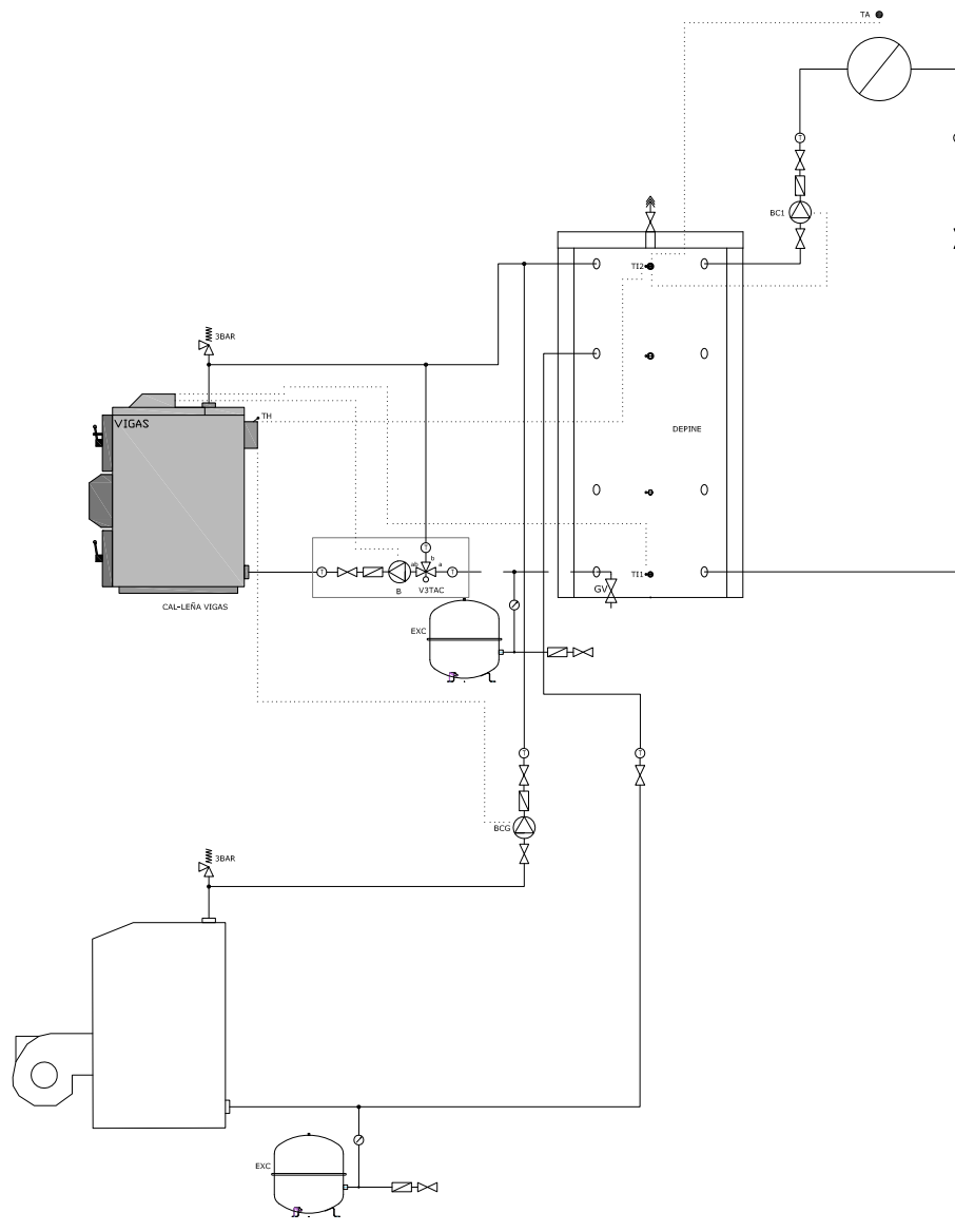
SOLO CALEFACCION CON GAS-GASOLEO E INERCIA
